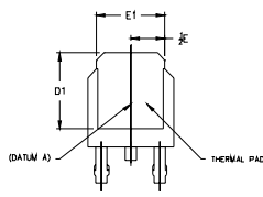
VIEW A-A
